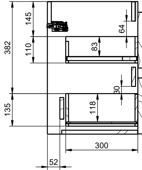
B-B ( 1 : 8 )
