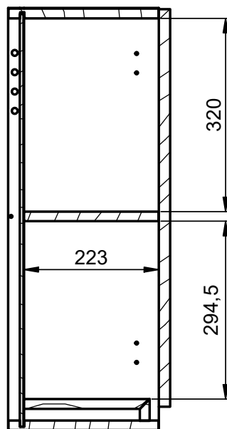
B-B ( 1:8 )
